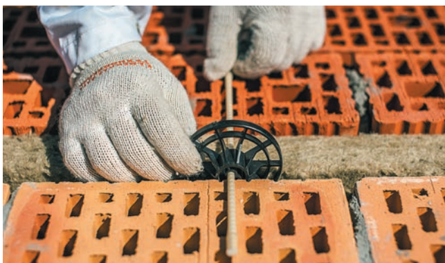
Рис. 13. Установка гибких связей
